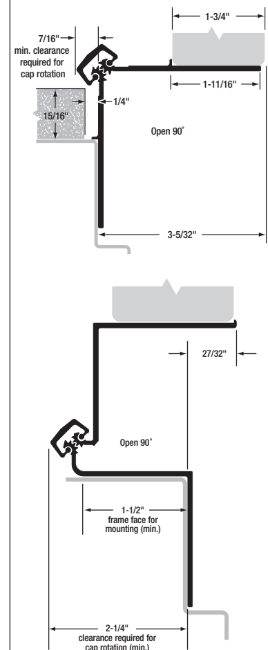
Fig. 2 Door Open 90°
