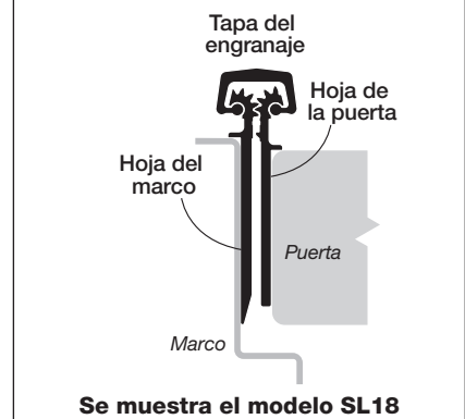
Fig. 2 Puerta abierta a 90°
