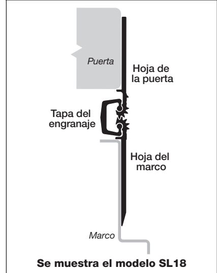
Fig. 3 Puerta abierta a 180°
